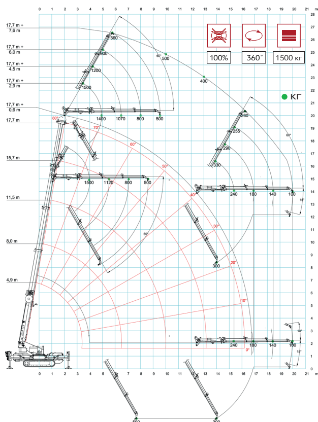
Гидравлический гусек JIB1500.3HL
