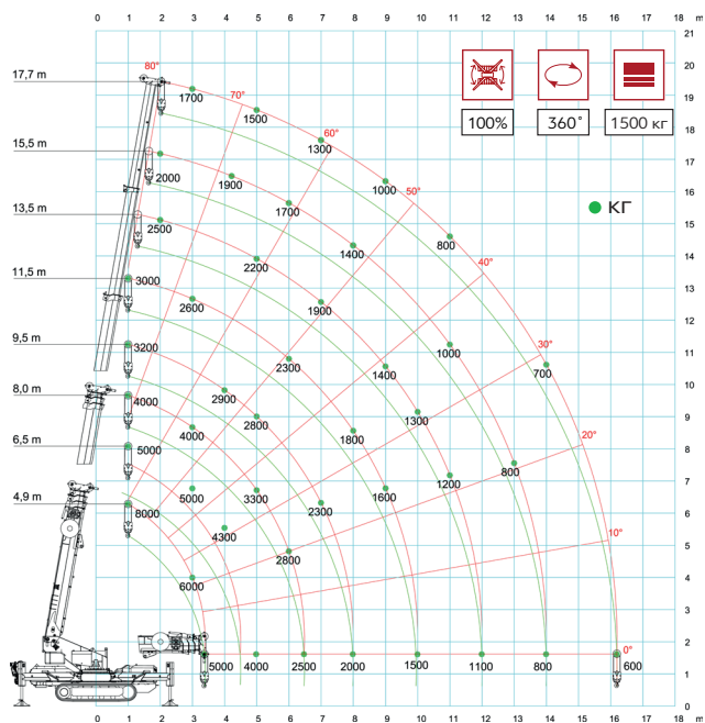
Основная стрела
