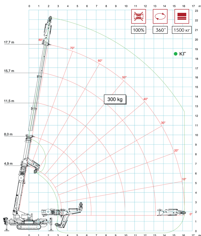
Граббер JIB300GR
